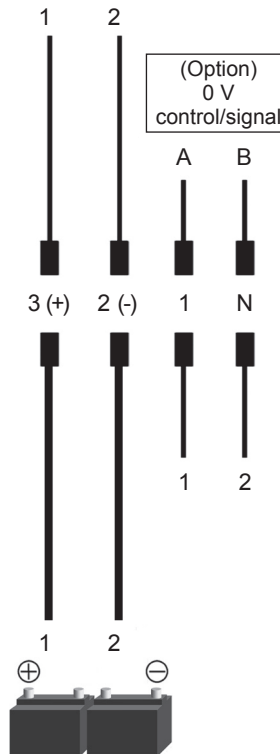
Rettbox® 20 A / 12/24 V
